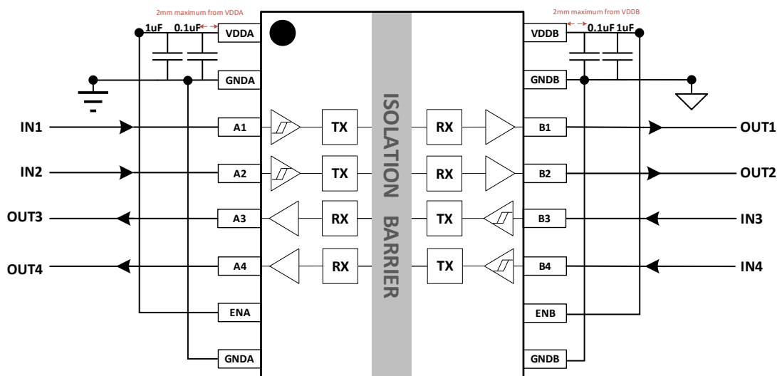
图 9-1 CA-IS3742C 典型应用电路
