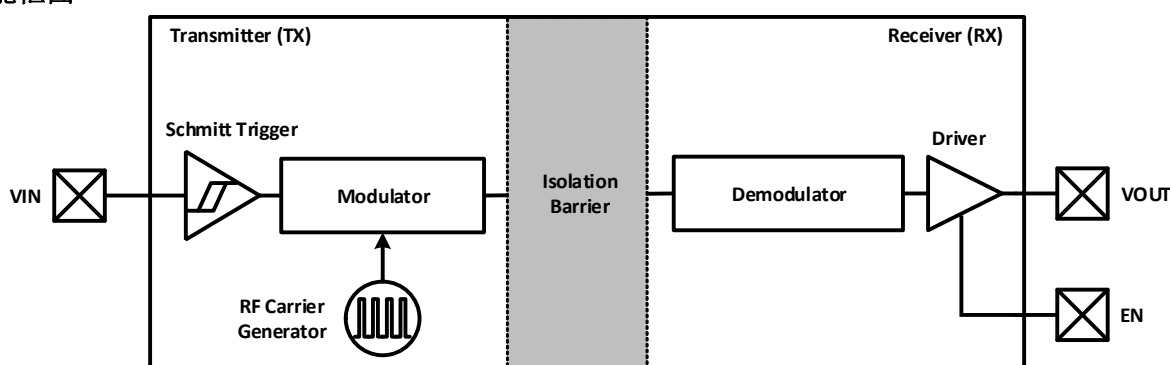
图 8-1 单通道功能框图
