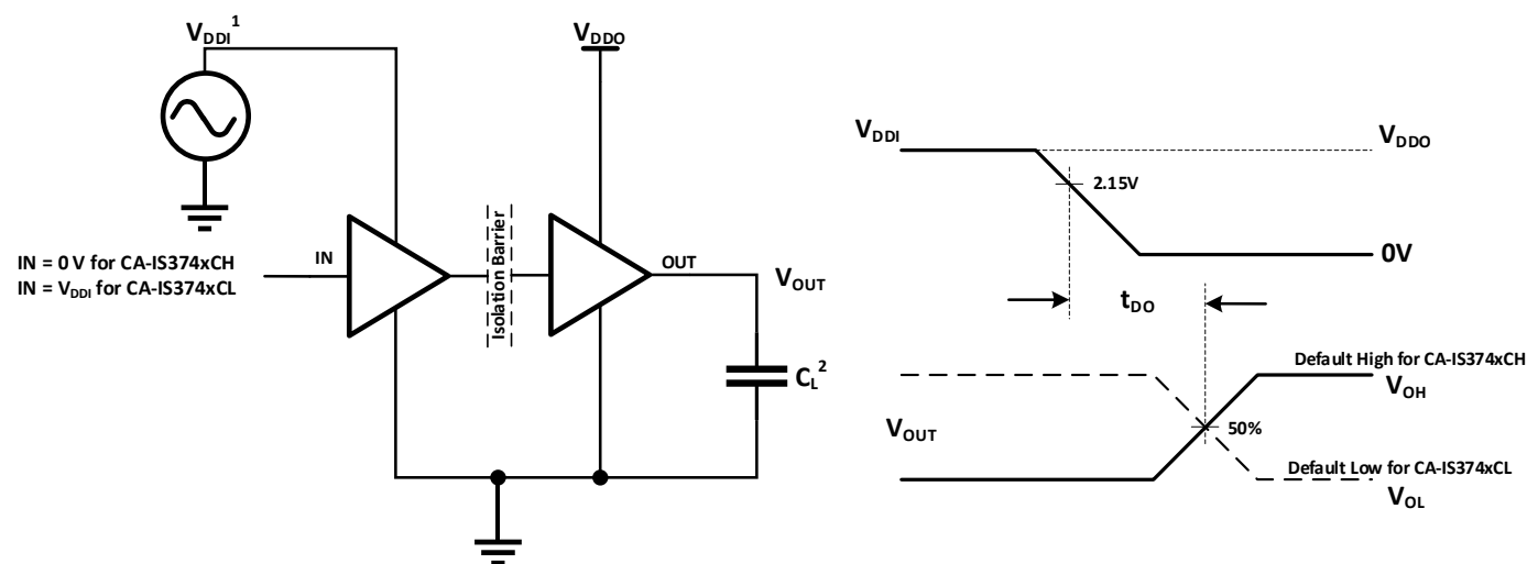
图 7-3 启用/禁用传播延迟时间测试电路和波形
