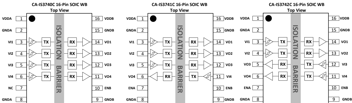
图 6-1 CA-IS374xC 顶部视图
